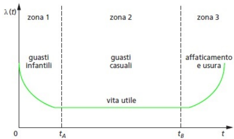
Curva “a vasca da bagno” (tecnica della manutenzione)
