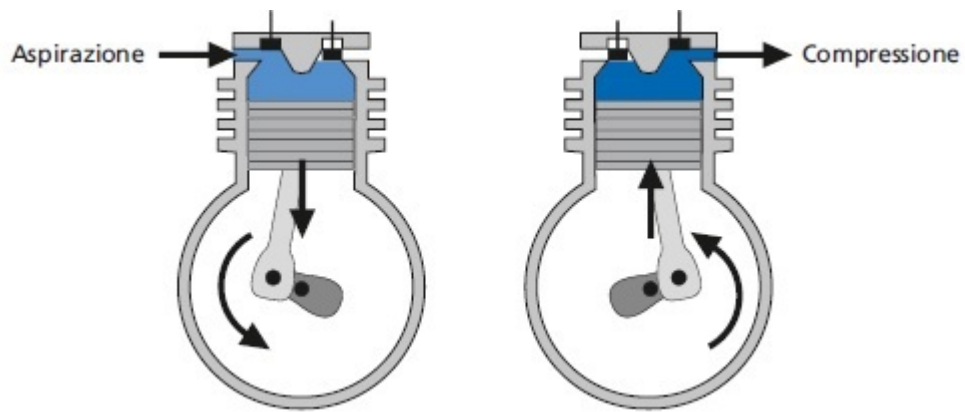
Compressore alternativo
